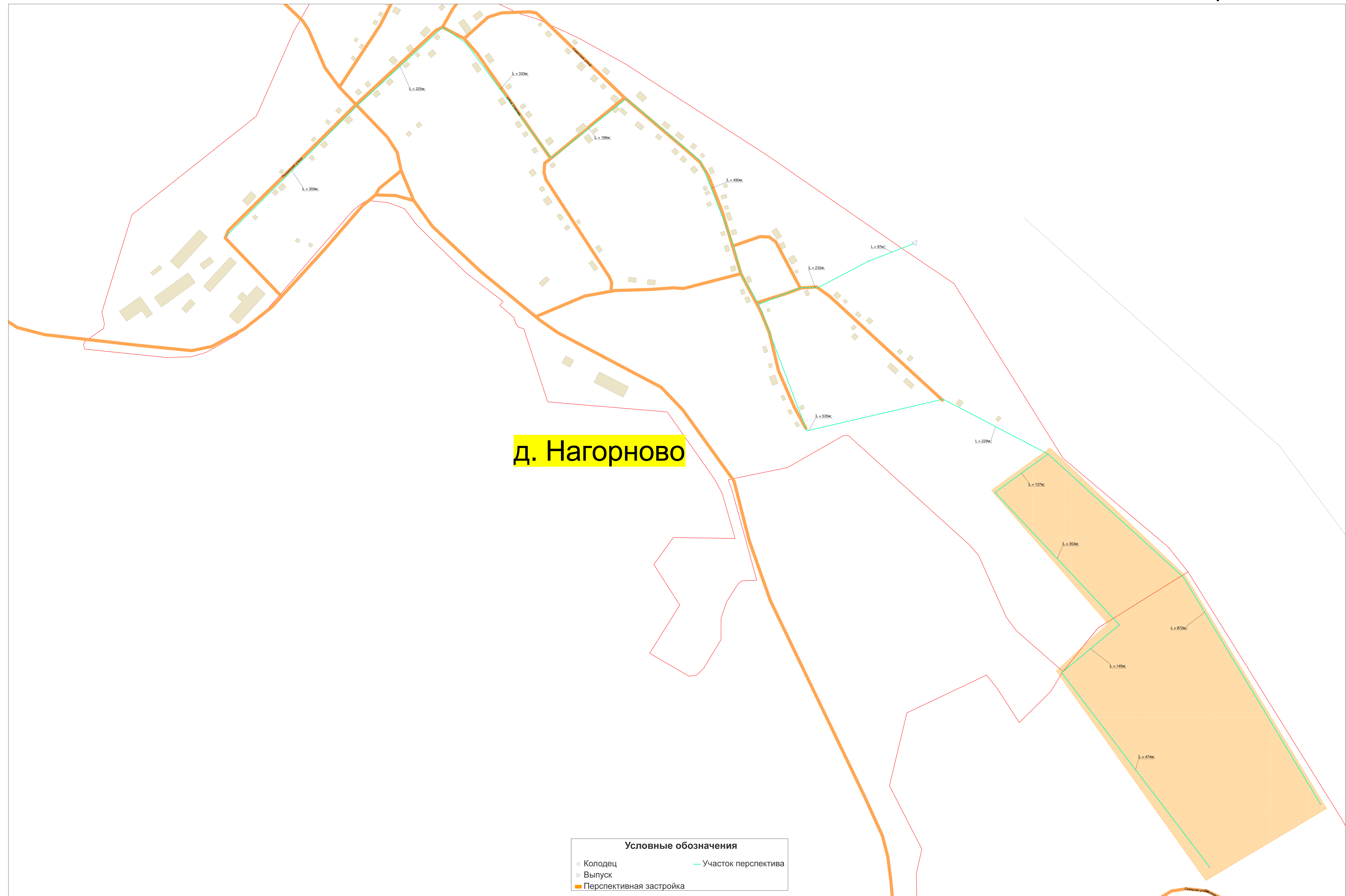
Рис. 2. Схема перспективного водоотведения д. Нагорново
