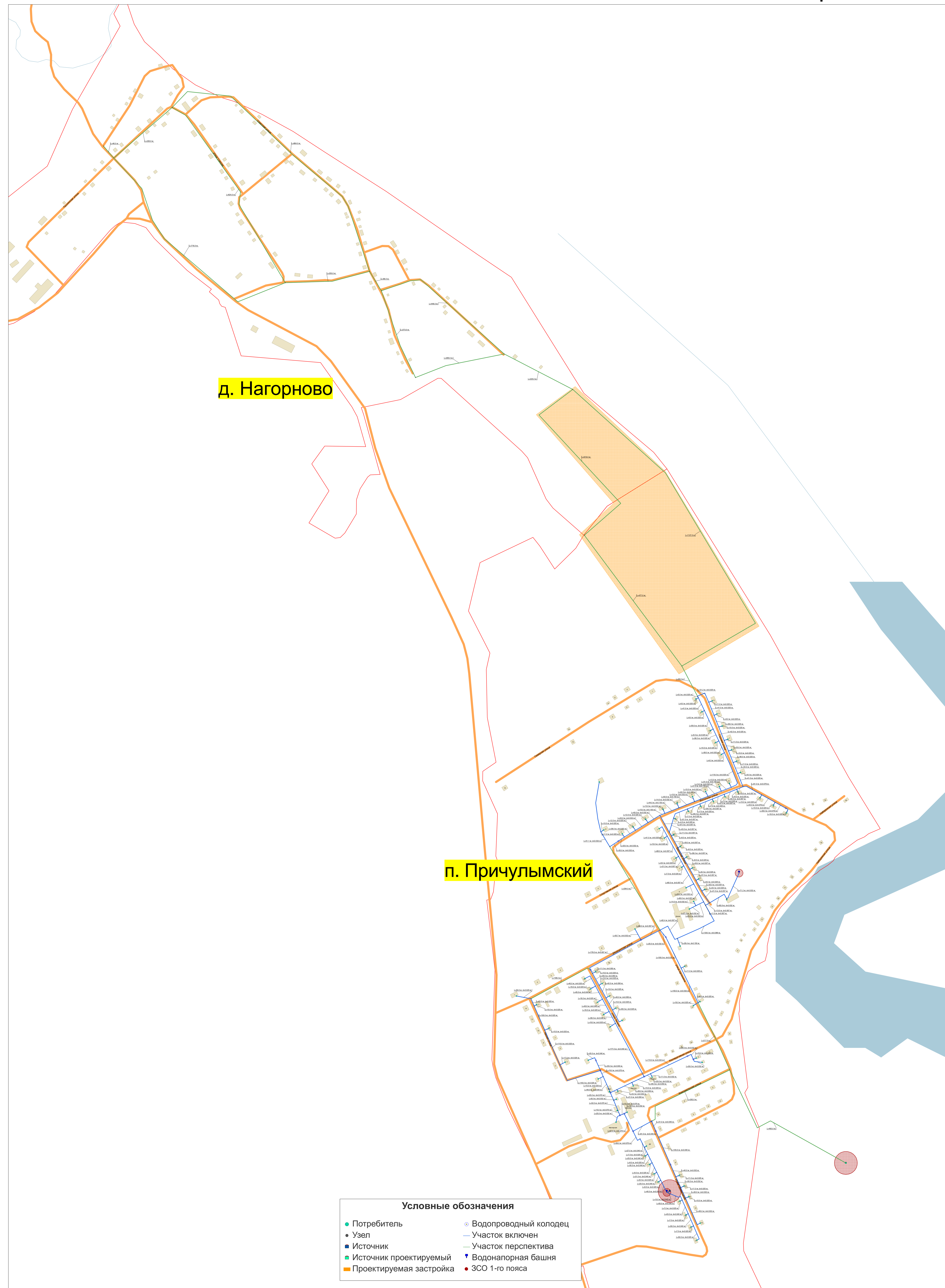
Рис. 3. Схема водоснабжения п. Причулымский и д. Нагорново
