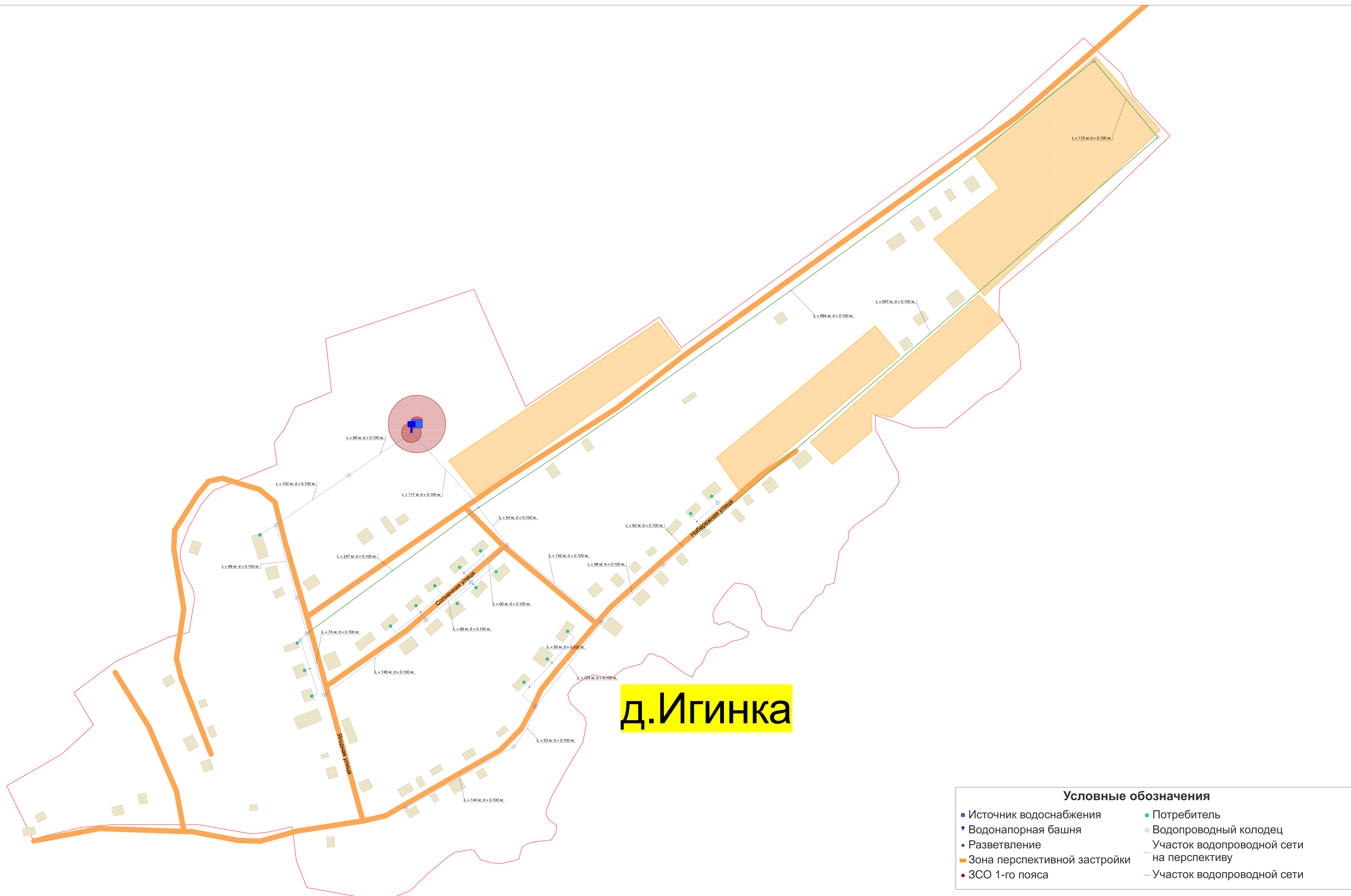
Рис. 3. Схема водоснабжения д.Игинка
