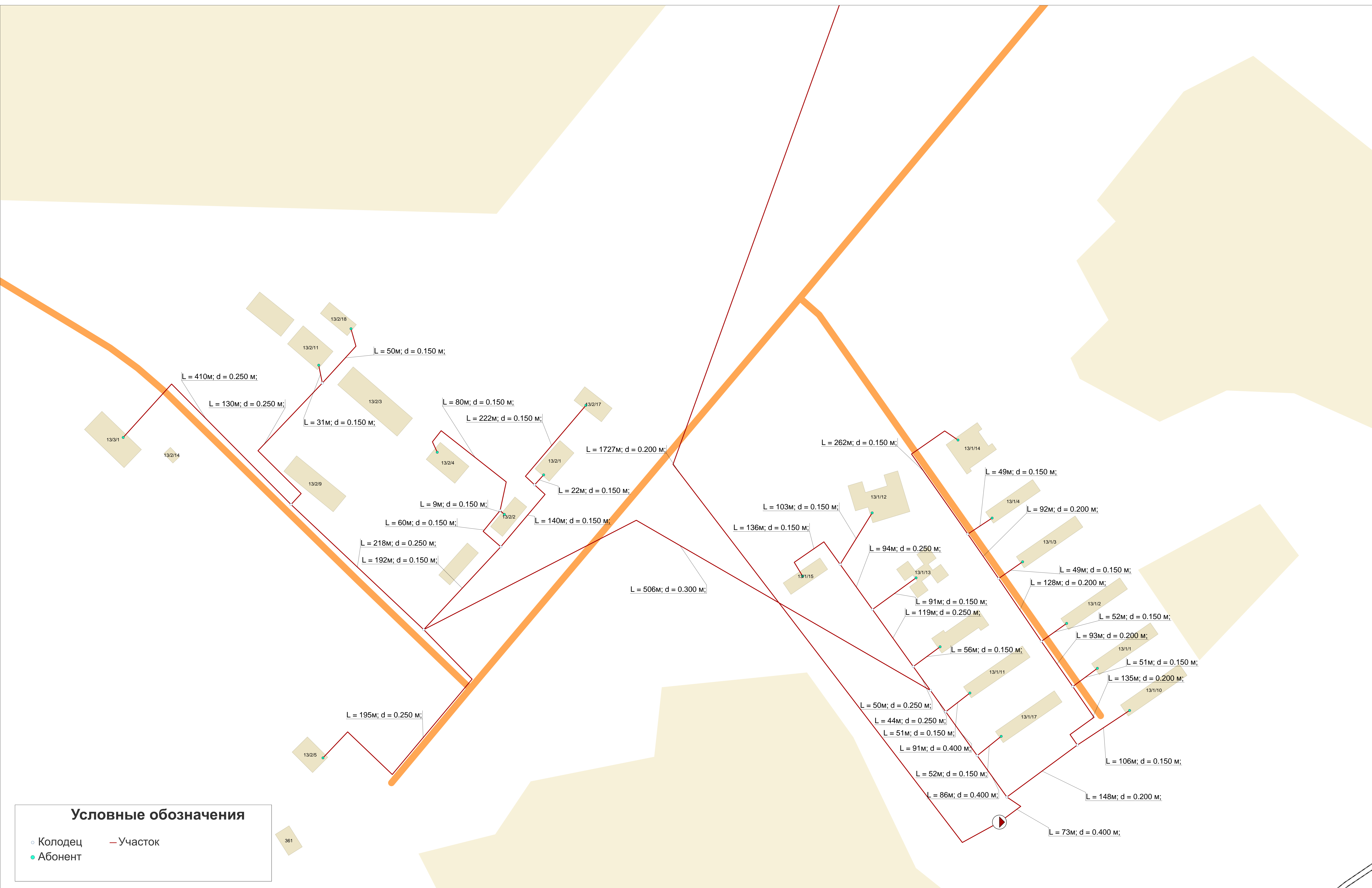
Рис. 9. Схема водоотведения военного городка №13 Участок №5
