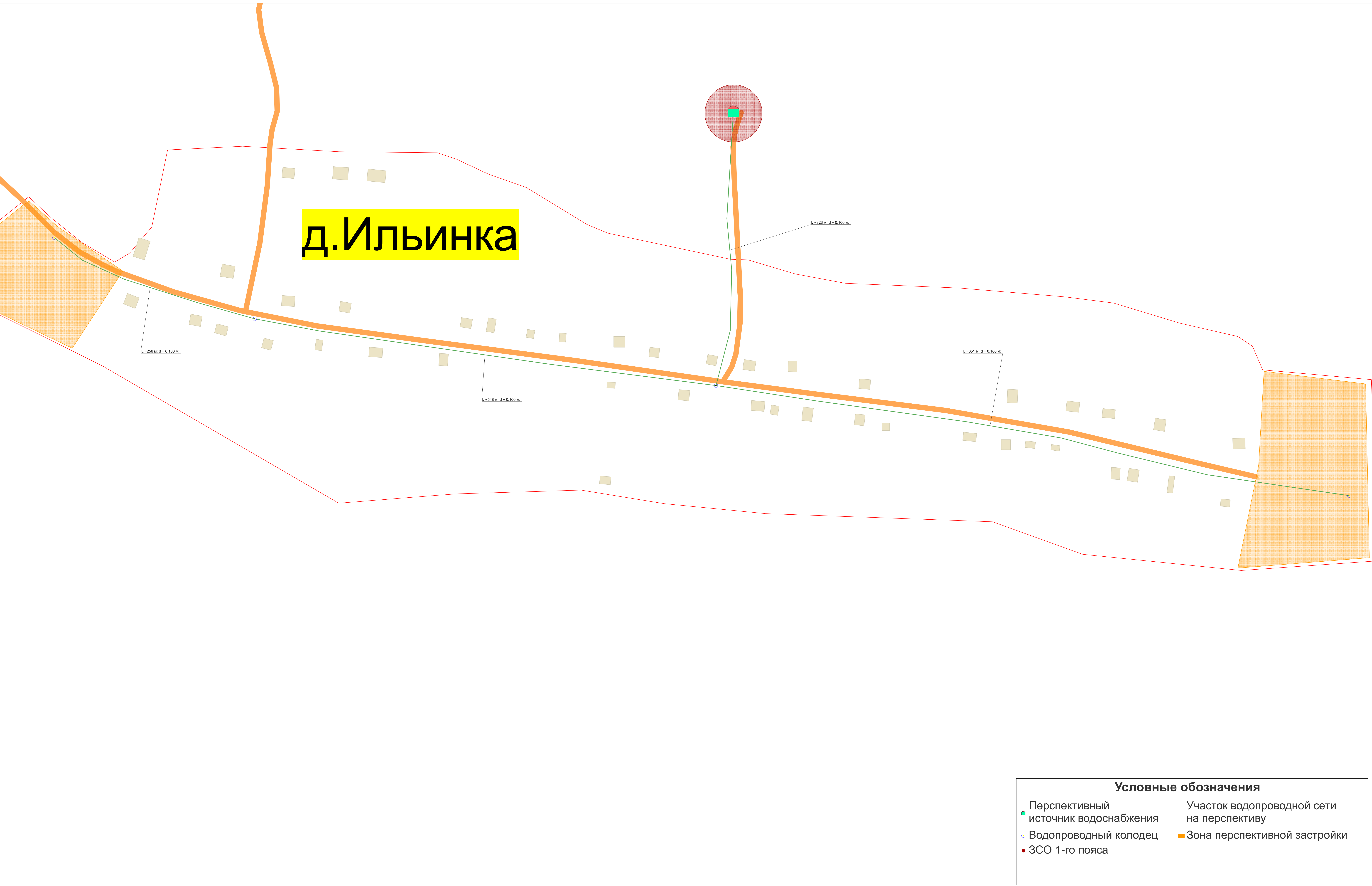
Рис. 2. Схема водоснабжения д.Ильинка
