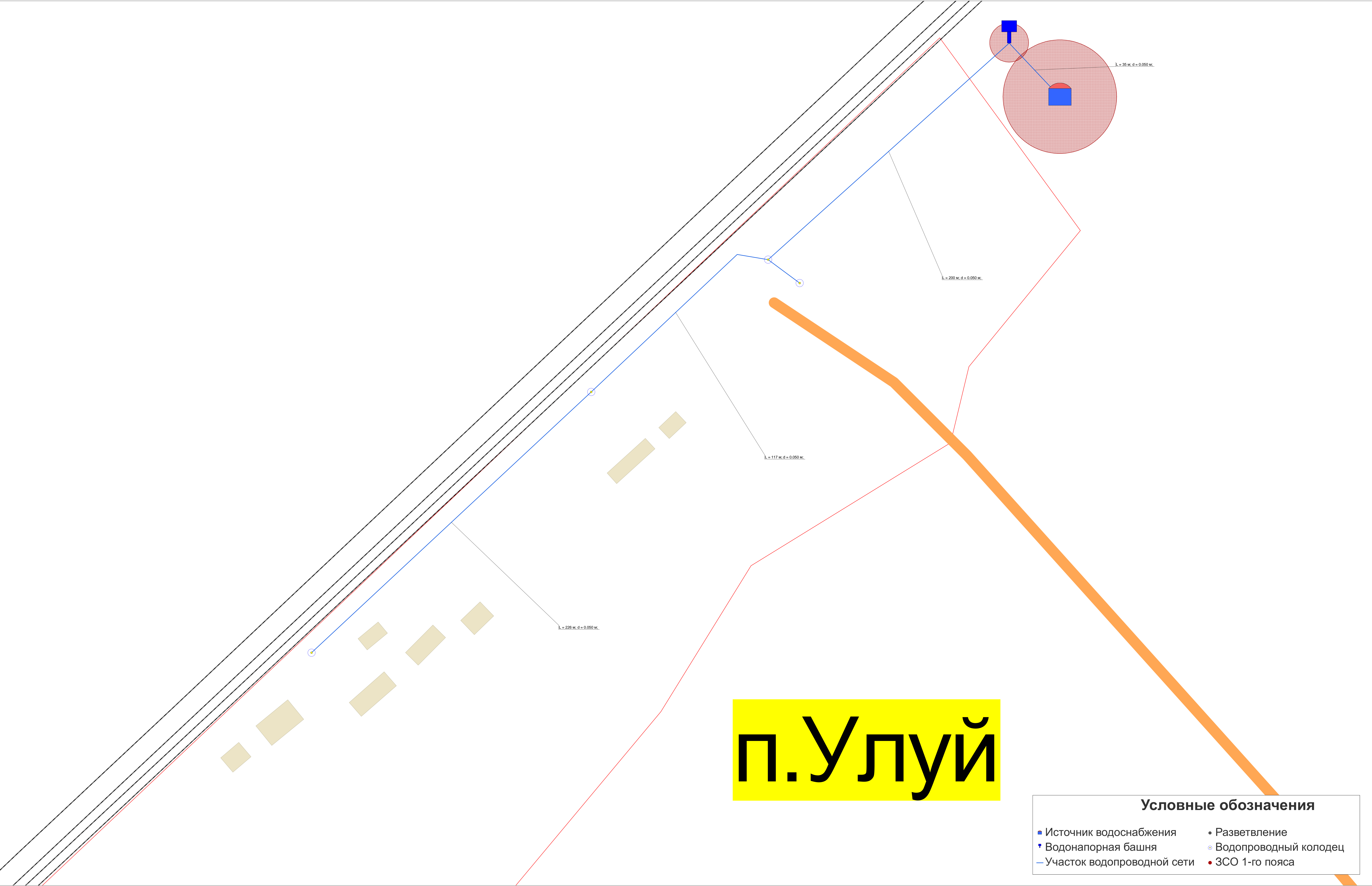
Рис. 3. Схема водоснабжения п.Улуй
